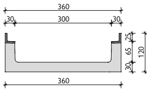
Gusszarge BH 120 mm
