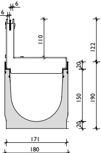
Schlitzaufsatz 2S, Heelproof SW 2x6, Kl. C
