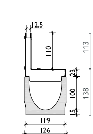
Schlitzaufsatz SW 12,5 Kl. C
