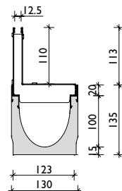
Schlitzaufsatz SW 12,5 Kl. C
