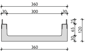
verzinkte Stahlzarge BH 120 mm
