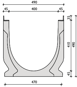
Gusszarge
