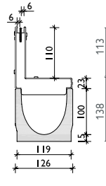
Schlitzaufsatz 2S, Heelproof SW 2x6, Kl. C
