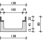
Gusszarge
