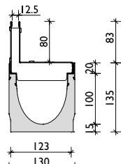
Schlitzaufsatz SW 12,5 Kl. B
