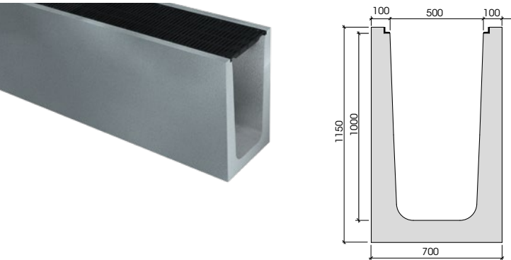
Gusszarge
