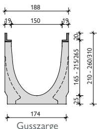
Gusszarge
