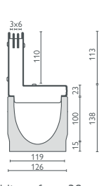
Schlitzaufsatz 3S, Heelproof SW 3x6, Kl. C
