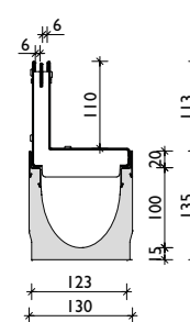
Schlitzaufsatz 2S, Heelproof SW 2x6, Kl. C
