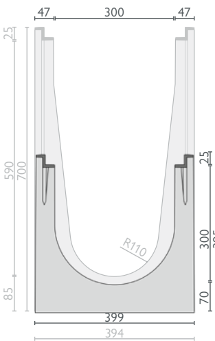
Gusszarge
