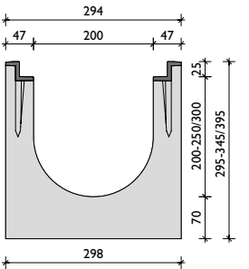
Gusszarge
