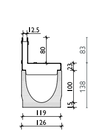
Schlitzaufsatz SW 12,5 Kl. B
