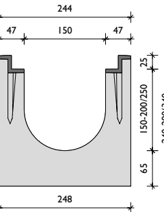
Gusszarge
