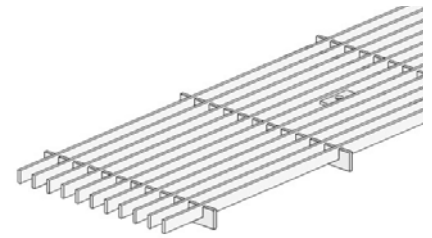
Längsstabrost 3 mm
